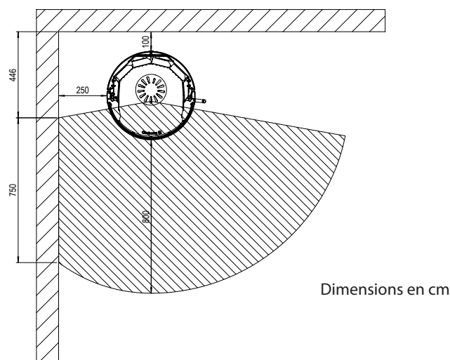
Poêle installé droit dans le coin
