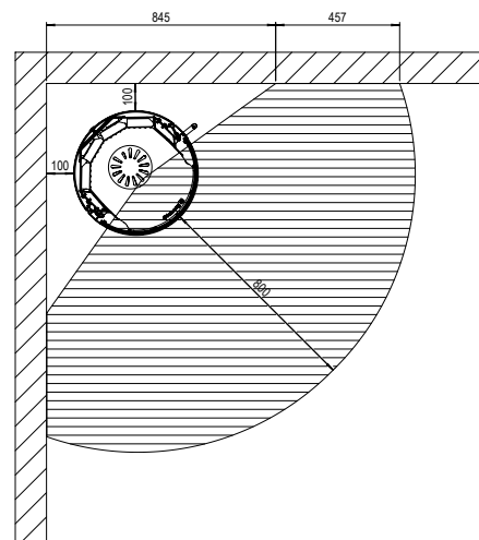
Kaminofen schräg in Ecke montiert (Abmessungen in cm)
