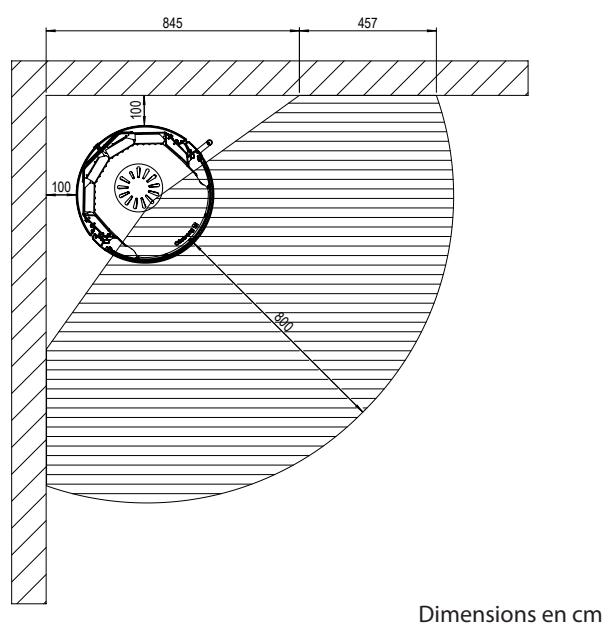
Poêle installé en biais dans le coin
