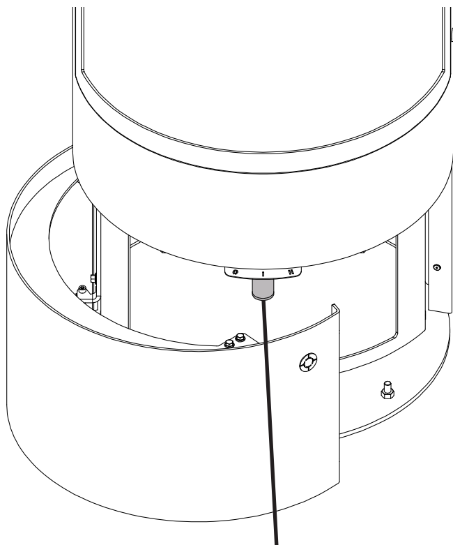
Lever de commande pour l'alimentation en air de combustion
