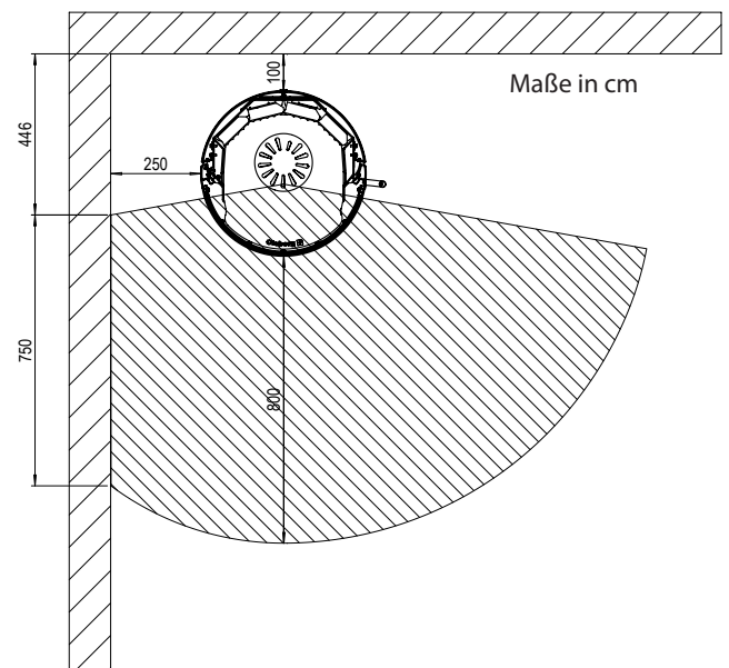
Kaminofen schräg in Ecke montiert
