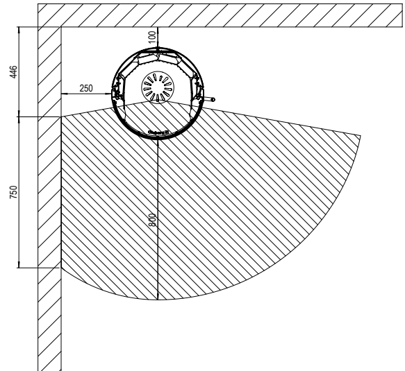
Kaminofen gerade in Ecke montiert.
