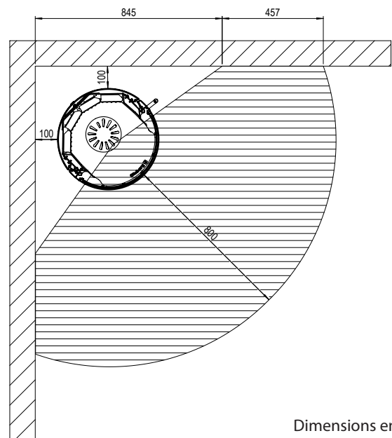
Poêle installé en biais dans le coin
